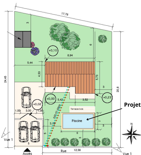
Plan de masse 1/200ème
